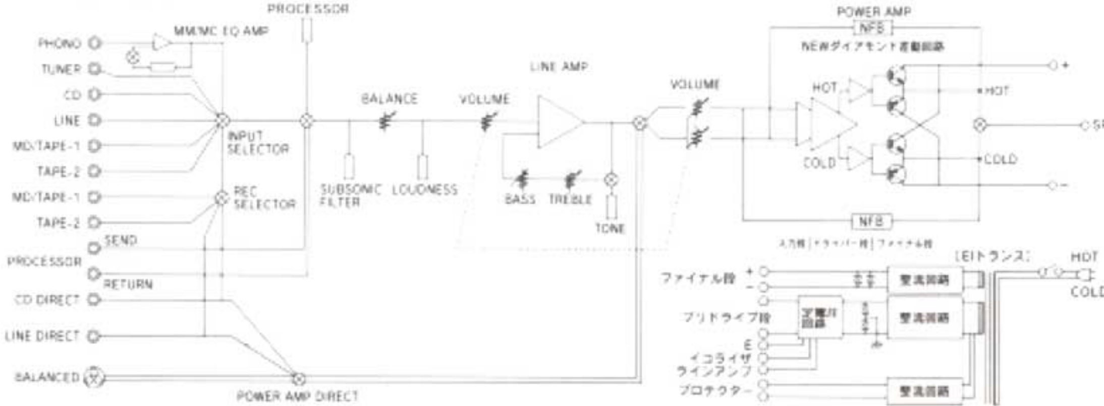
ブロックダイアグラム
