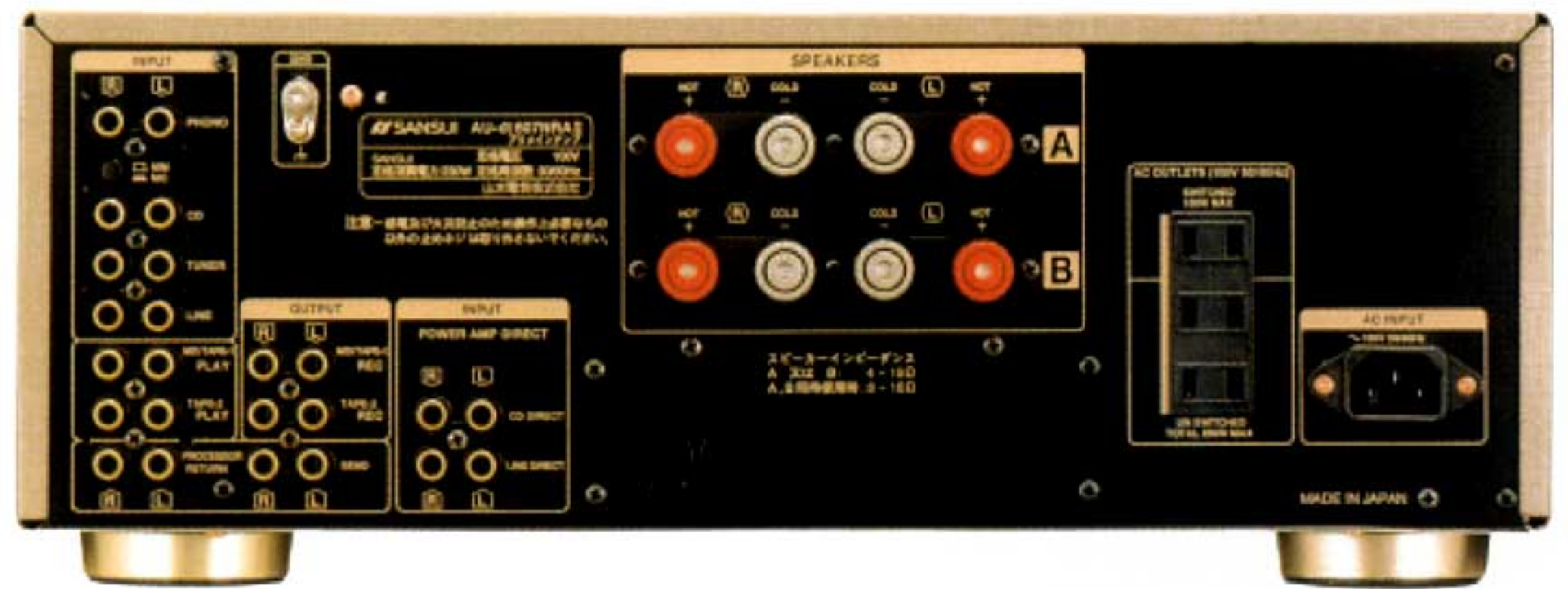
オール金メッキ入力端子を装着したリアパネルレイアウト
